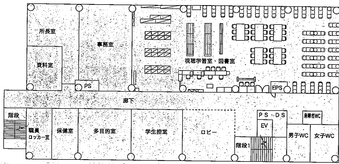
5階平面図
