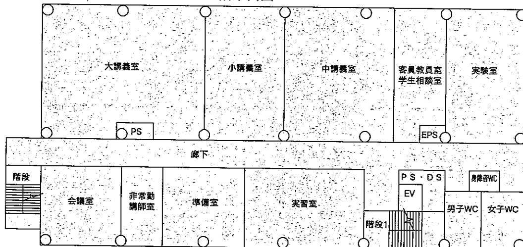
6階平面図
